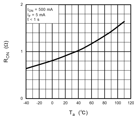
Fig. 14.1.5 R_{ON} - T_a
