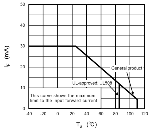
Fig. 14.1.1 I_F - T_a
