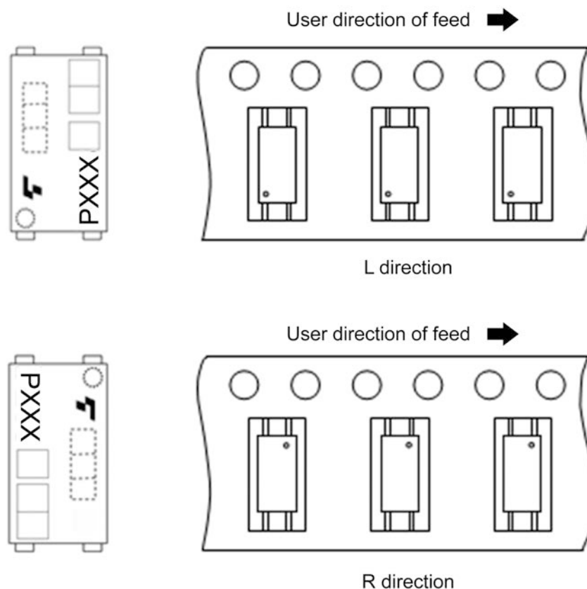
Fig. 16.3.1.1 Device Orientation
