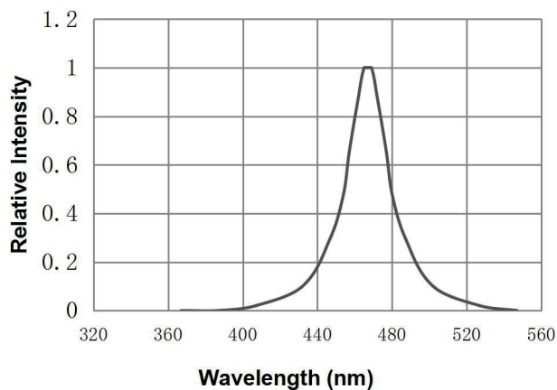
光谱分布特性曲线 Spectrum Distribution ( T_a=25^\circ\text{C} )
