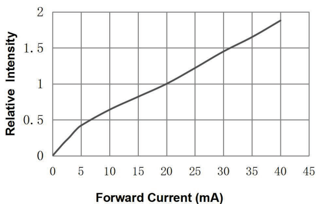
相对光强与电流特性曲线 Relative Intensity VS. Forward Current ( T_a=25^\circ\text{C} )
