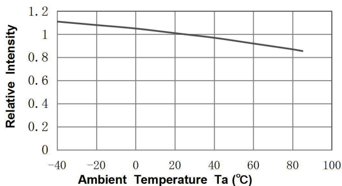
相对光强与环境温度特性曲线 Relative Intensity VS. Ambient Temperature ( T_a=25^\circ\text{C} )
