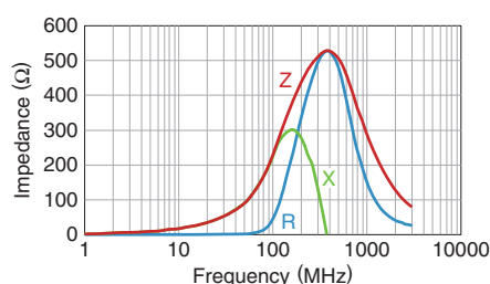
MMZ1608Q221BTA00
