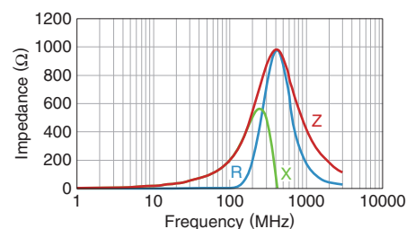
MMZ1608D241CTA00
