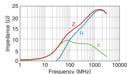
MMZ1608Y150BTA00
