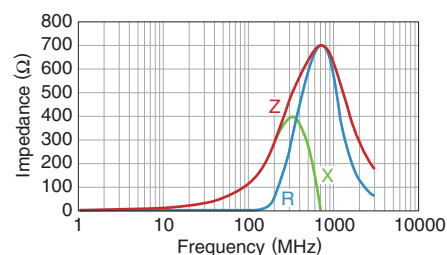
MMZ1608D121CTAH0
