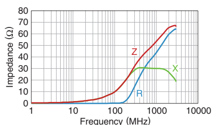
MMZ1608D800CTAH0
