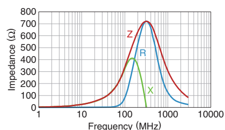
MMZ1608Q331BTA00
