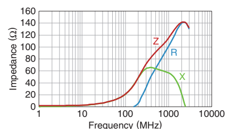
MMZ1608D800BTA00
