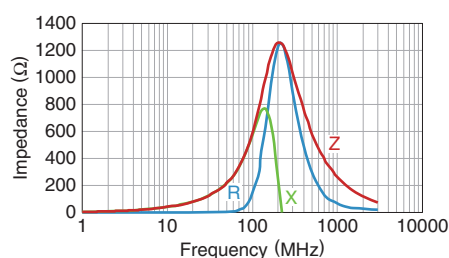
MMZ1608Q601BTA00
