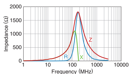
MMZ1608Q102BTA00
