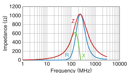
MMZ1608Q471BTA00
