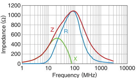
MMZ2012S102AT000
